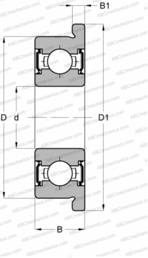
РАЗМЕРЫ, ММ
